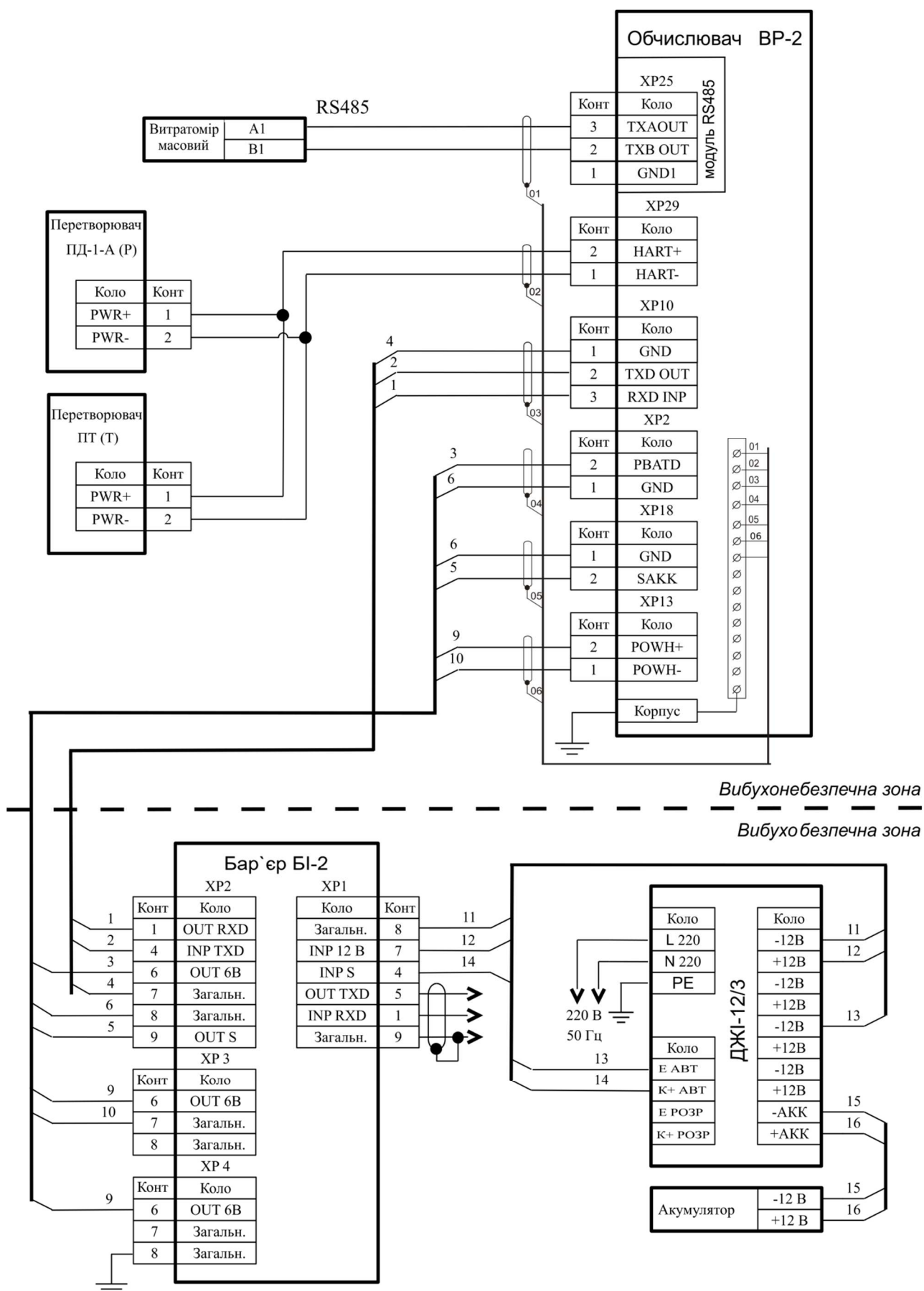
Рис. В.14 - Схема підключення масового витратомірів до обчислювача ВР-2 у складі одноканального Комплексу «ФЛОУТЕК-ТМ-1-4-1»). Дані про витрату середовища передаються від витратомірів по інтерфейсу RS485. Обчислювач розміщується у вибухобезпечній зоні.
