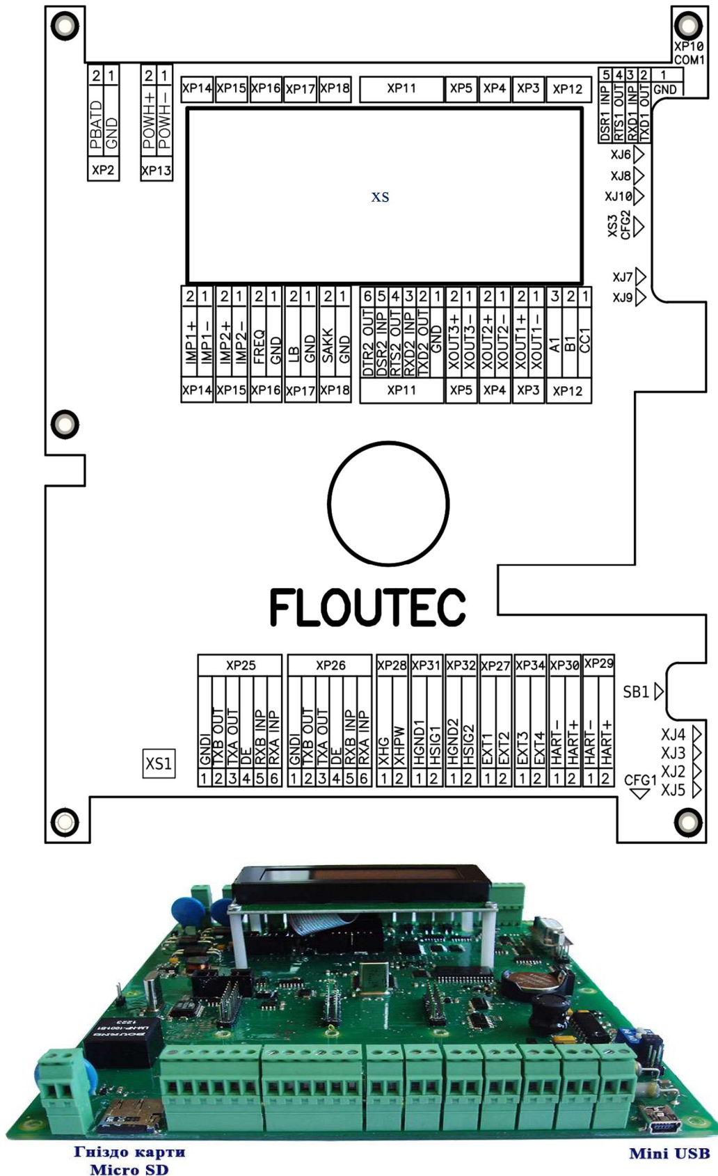
Рис. Б.1 – Фальш-панель захисту елементів плати Обчислювача ВР-2 та розміщення гнізд зовнішніх підключень.
