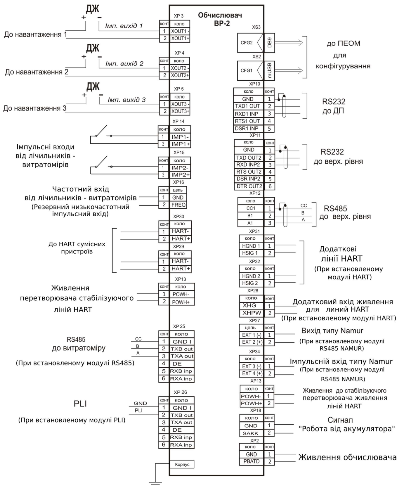
Рис. А.1– Схема зовнішніх з'єднань Обчислювача ВР-2 з пристроями у складі комплексу «ФЛОУТЕК–ТМ»
