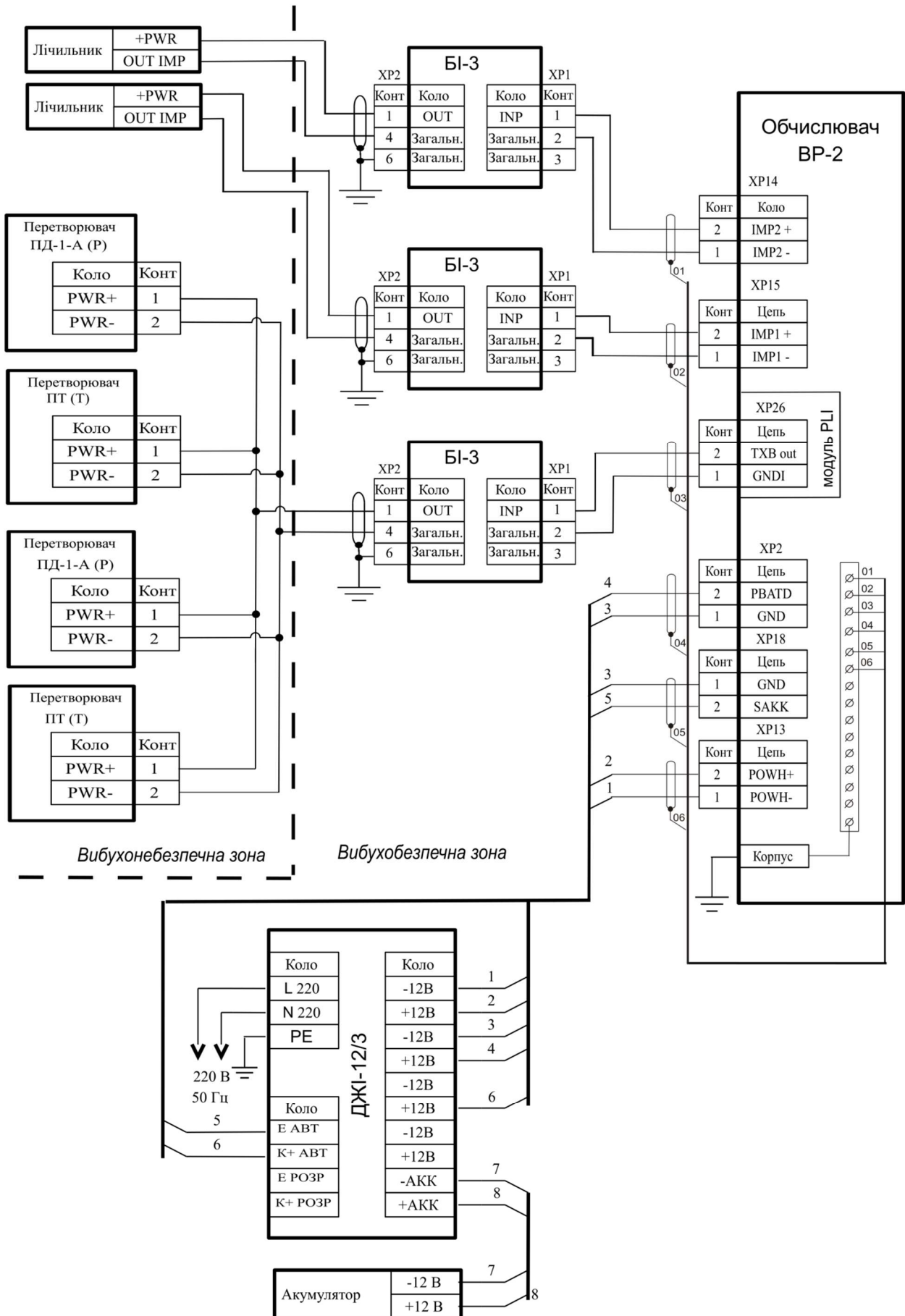
Рис. В.2 – Схема підключення Обчислювача ВР-2 у складі двоканального комплексу «ФЛОУТЕК-ТМ-1-33-11». (Витратоміри з імпульсним вихідним сигналом. Обчислювач розміщується поза вибухонебезпечної зони. Встановлено додатково модуль PLI)
