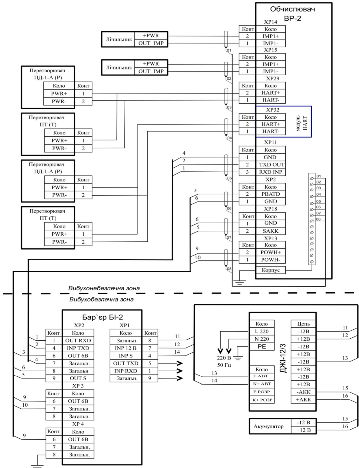
Рис. В.1 – Схема підключення Обчислювача ВР-2 у складі двоканального комплексу «ФЛОУТЕК-ТМ-1-33-11». (Витратоміри з імпульсним вихідним сигналом. Обчислювач розміщується у вибухонебезпечній зоні. Встановлено додатково модуль Bell202)
