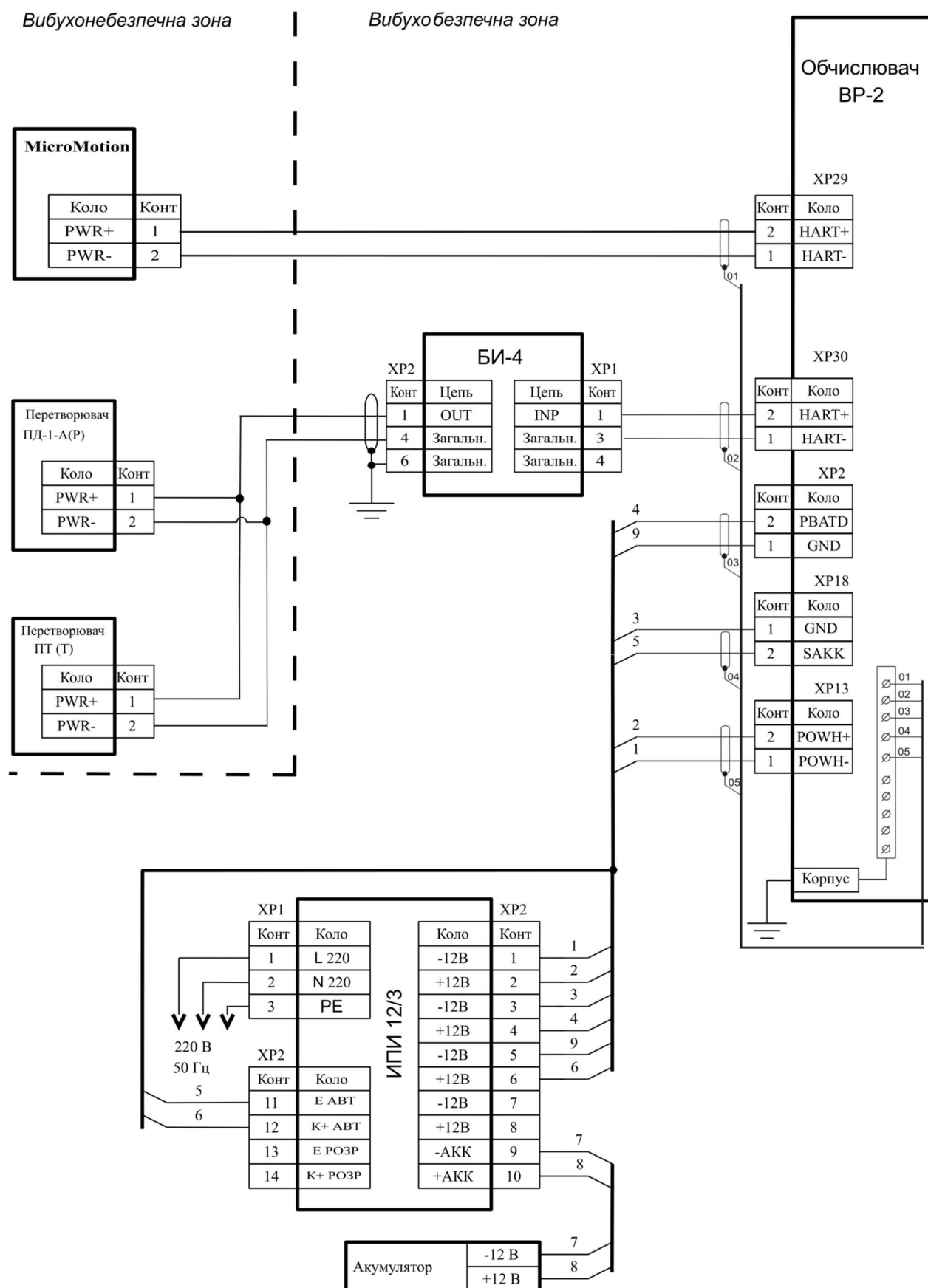
Рис. В.12 - Схема підключення витратоміра MicroMotion до обчислювача ВР-2 у складі одноканального Комплексу «ФЛОУТЕК-ТМ-1-4-1»). Дані про витрату середовища передаються від витратоміру по інтерфейсу HART. Обчислювач розміщується у вибухобезпечній зоні
