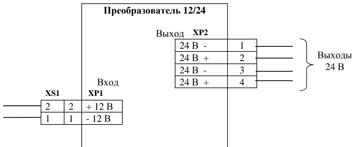
Рис. 1 Схема подключения преобразователя 12/24
